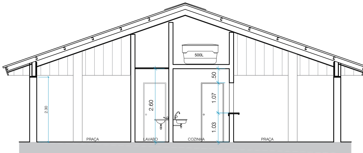
CORTE AA QUIOSQUE ESCALA: 1/50
